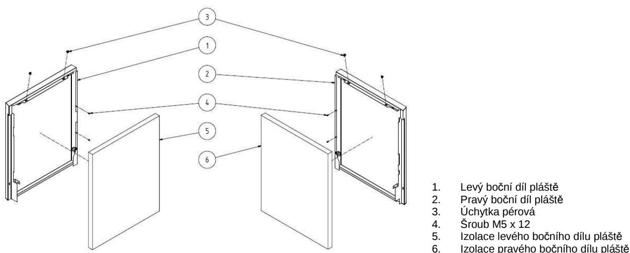
Obr. č. 16 Boční díly pláště
