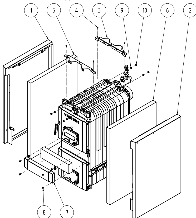
Obr. č. 17 Montáž bočních dílů pláště
